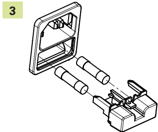
ヒューズホルダとヒューズ
