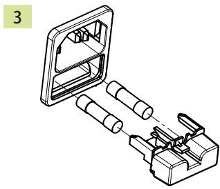
保險絲座與保險絲
