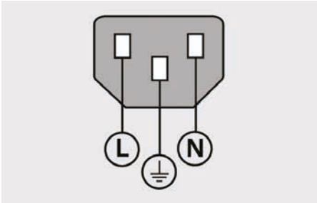
电源线
