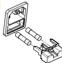
Portafusibles y fusibles
