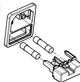
Suporte para fusível e fusíveis
