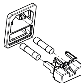
Кассета предохранителя и предохранители
