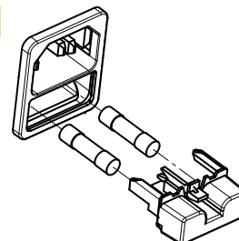
Portafusibili e fusibili
