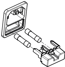
保险丝座和保险丝
