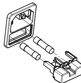
Držák pojistky a pojistky
