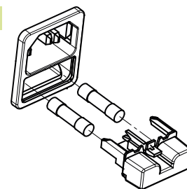
Fusibles et porte-fusible
