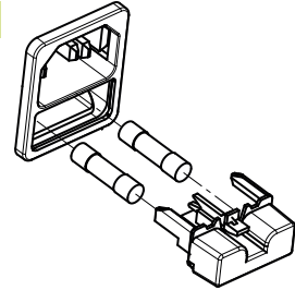
Sigorta yuvası ve sigortalar
