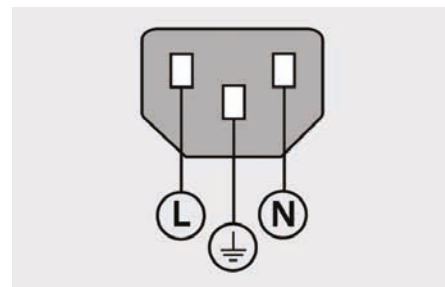
Netzkabel
