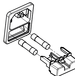
Sicherungshalterung und Sicherung
